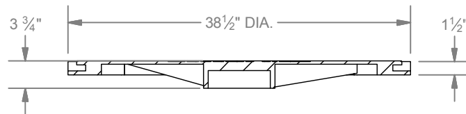
SECTION A-A SCALE 1:15
