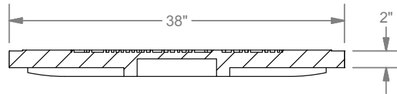
SECTION A-A SCALE 1:15
